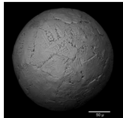
Fig. 10. Magnetite spherule.
